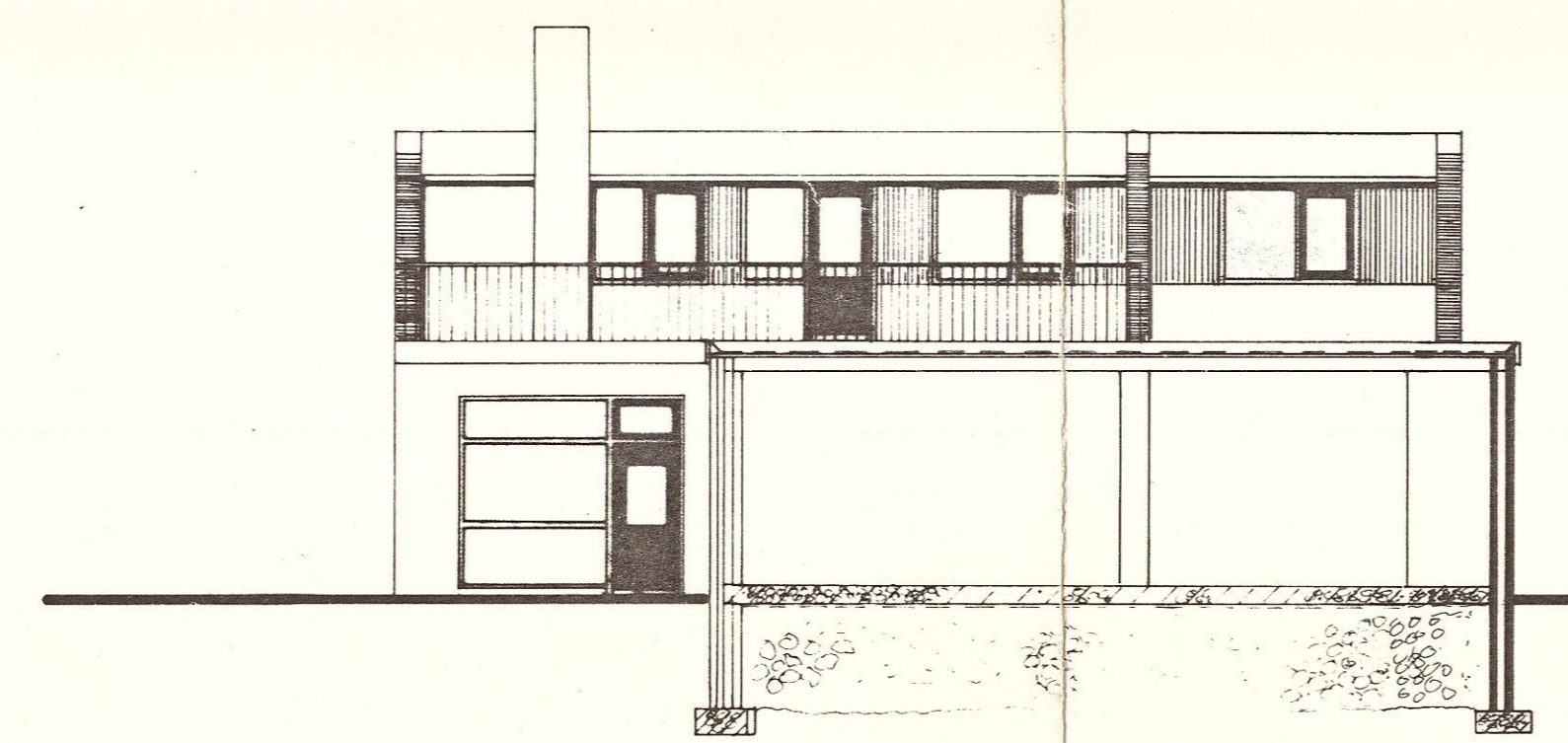
Achtergevel+doorsnede A-B
