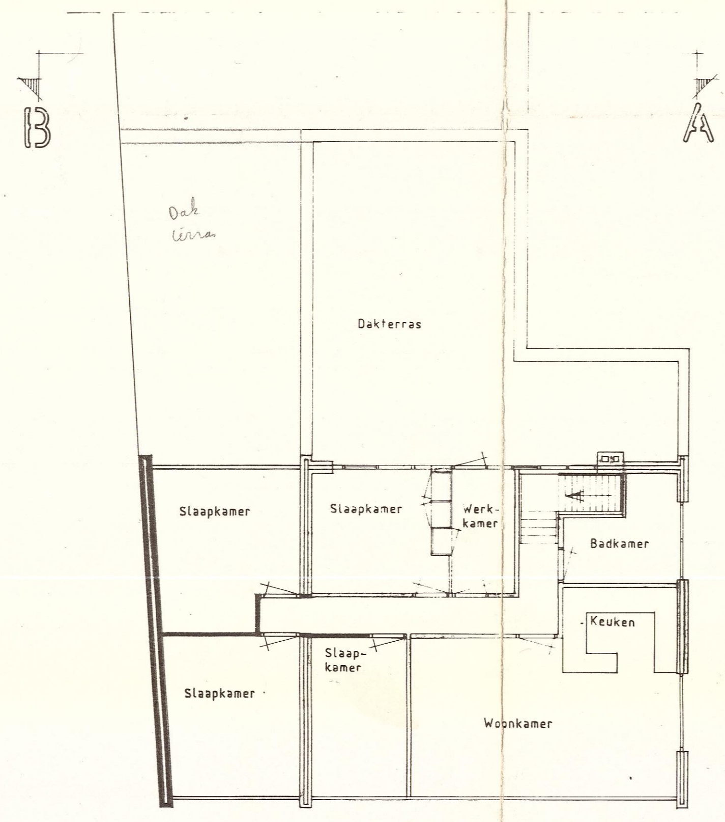
Verdieping
