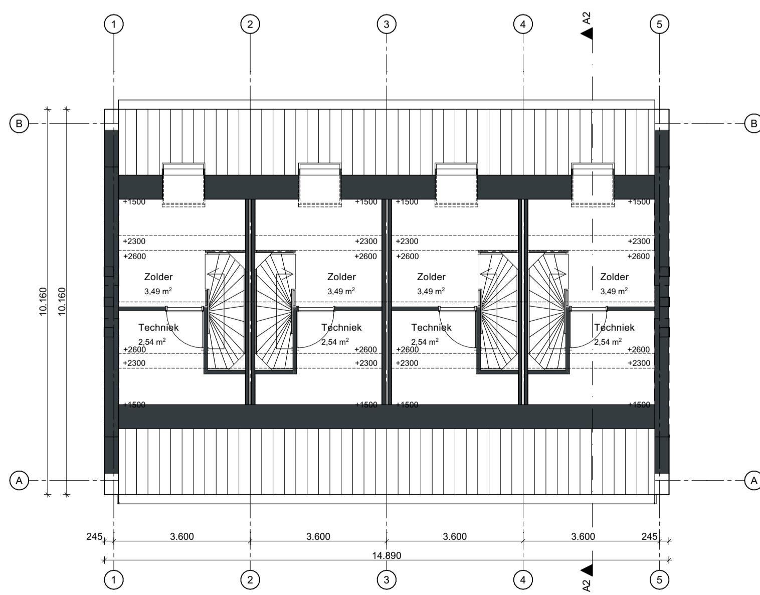
02 tweede verdieping
