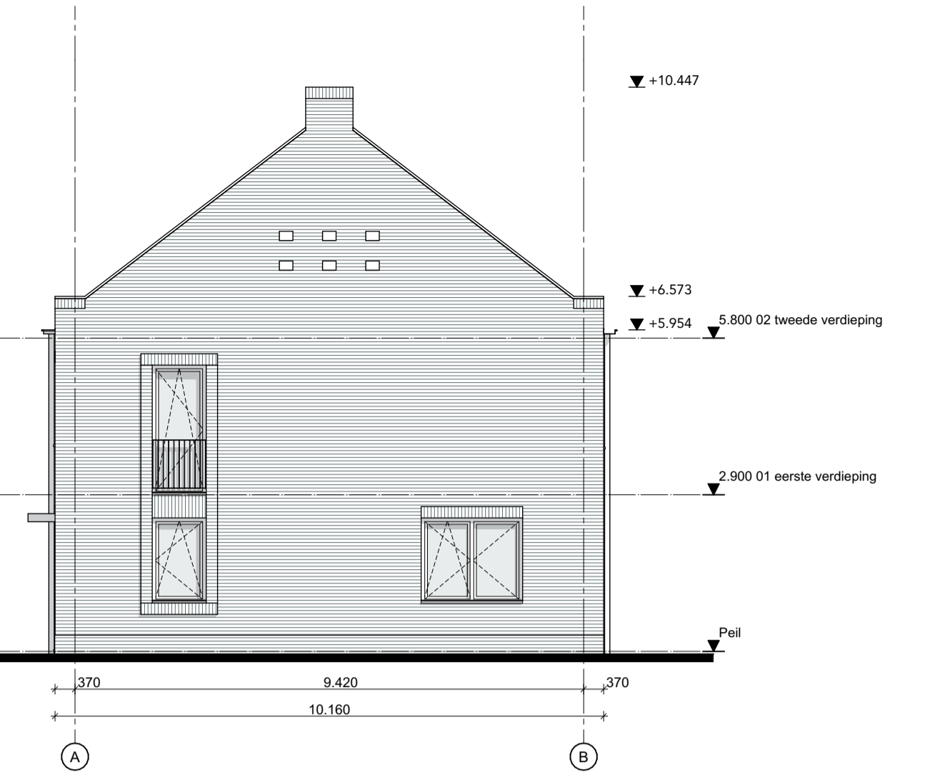
Rechtergevel
