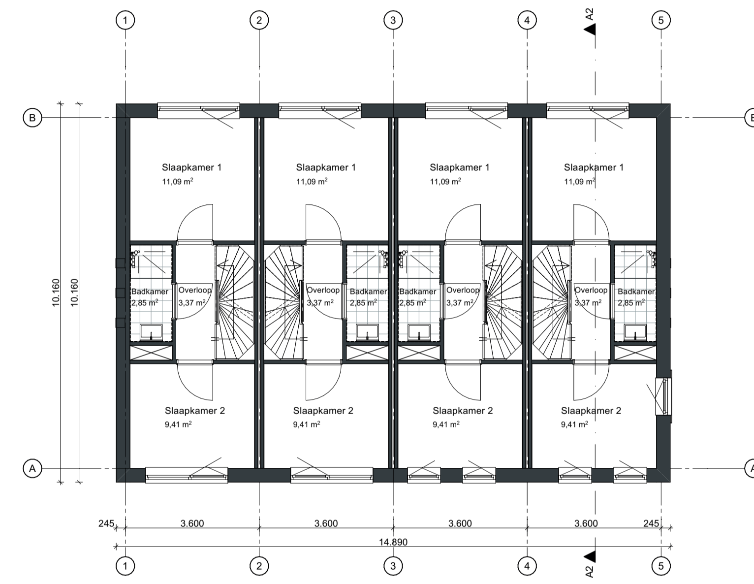
01 eerste verdieping
