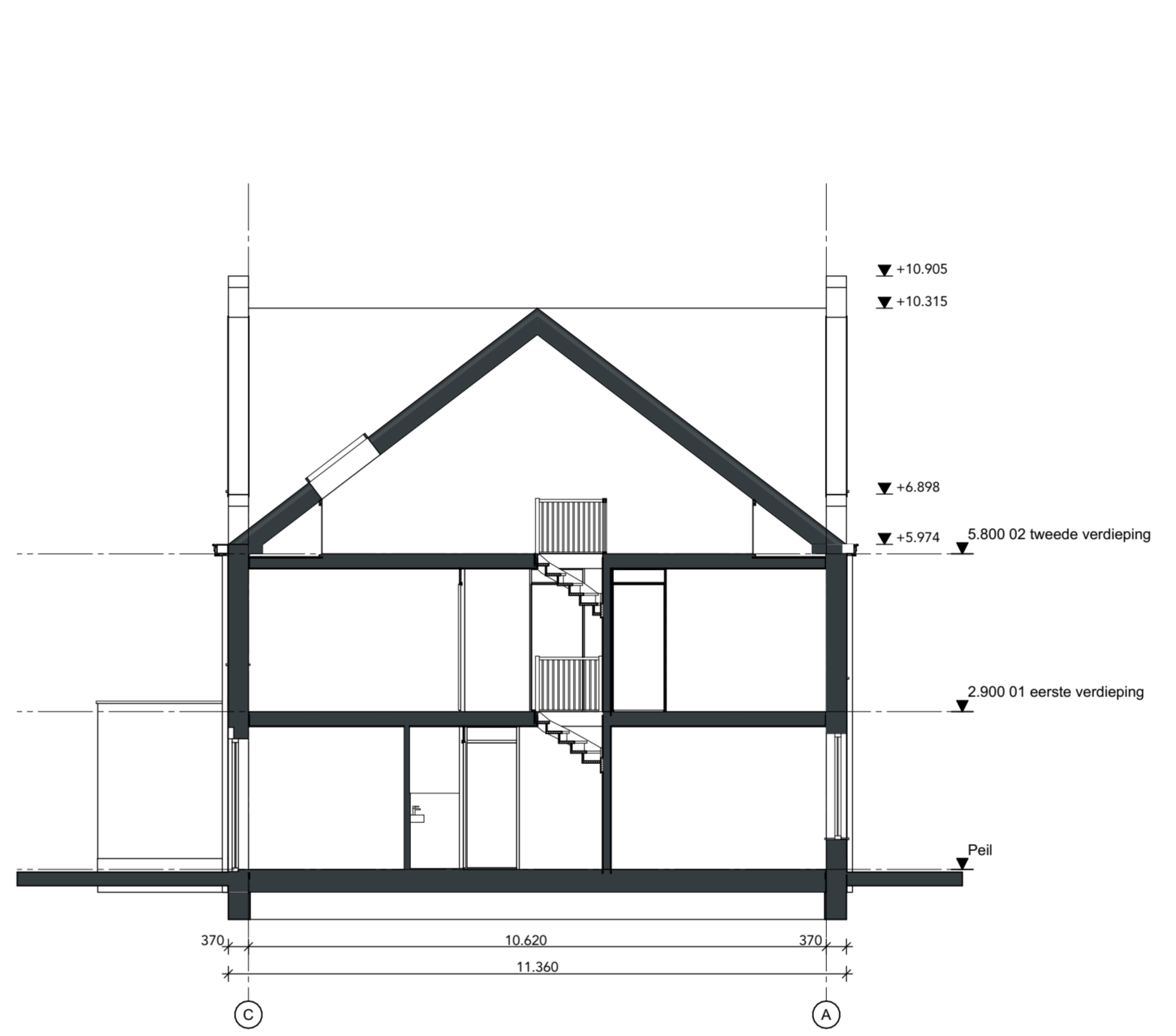
Doorsnede A-A
