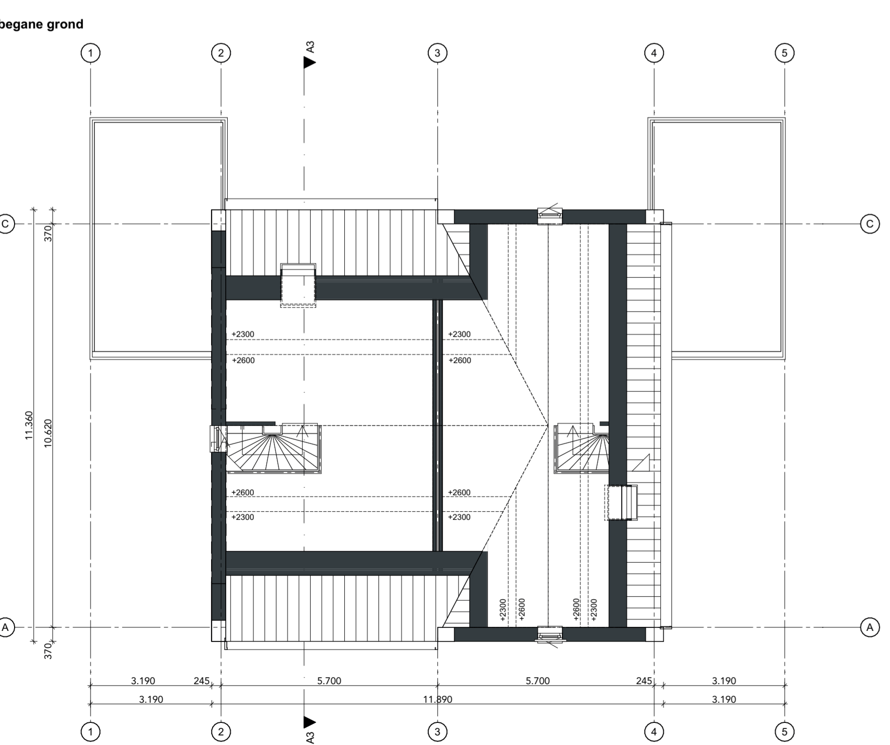
02 tweede verdieping
