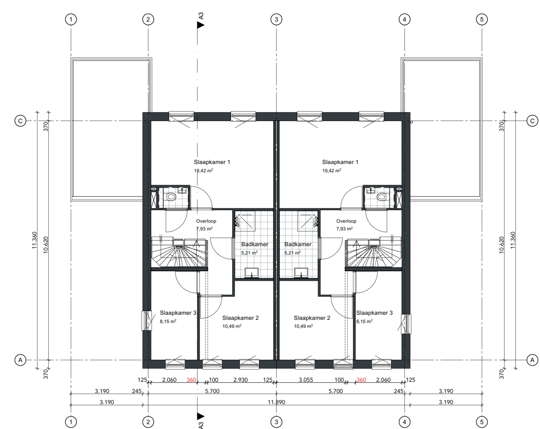
01 eerste verdieping
