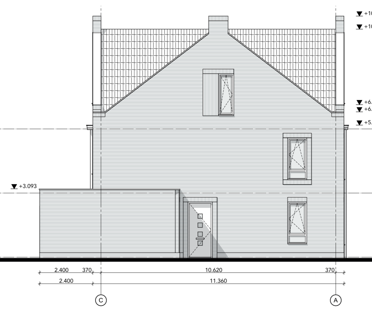
Linkergevel
