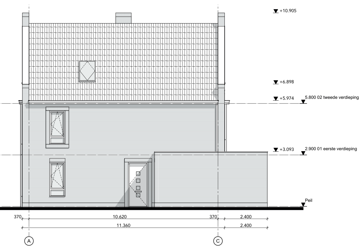
Rechtergevel
