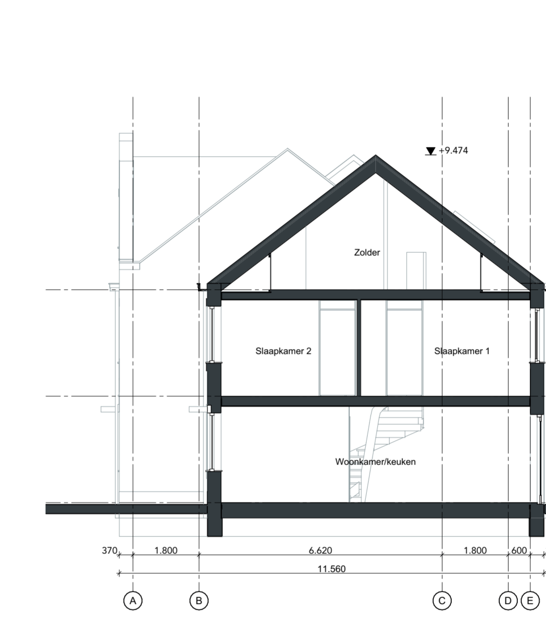
Doorsnede A-A
