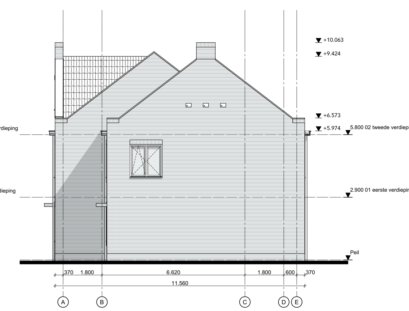
Rechtergevel
