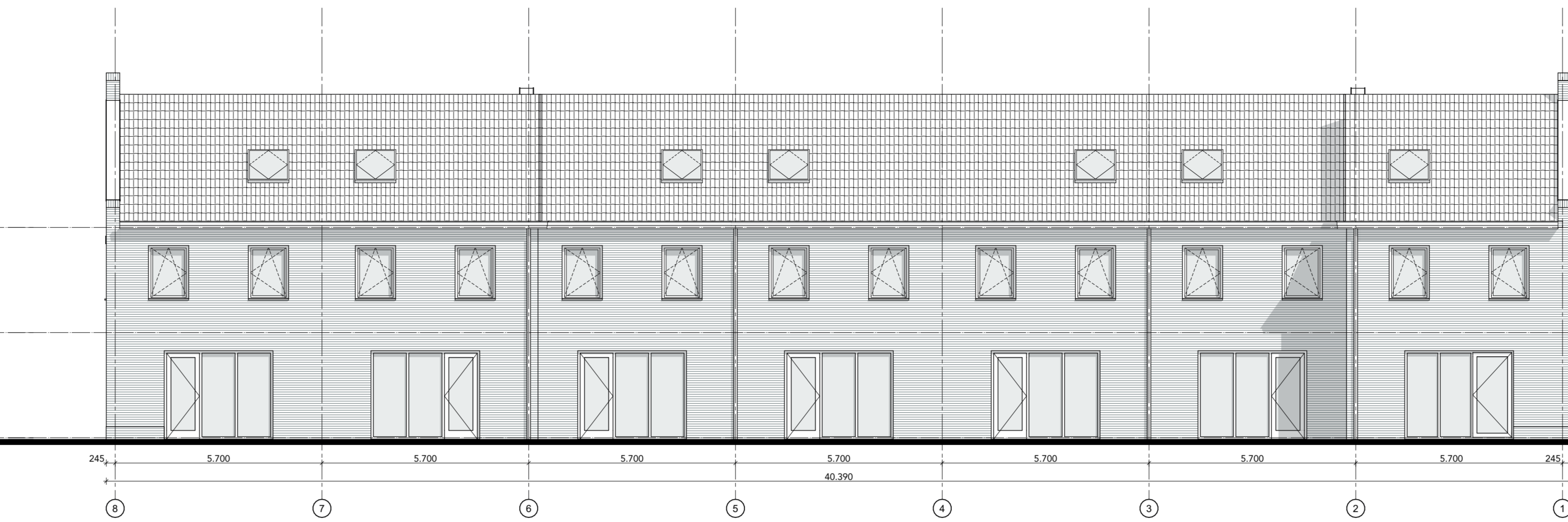
Achtergevel
