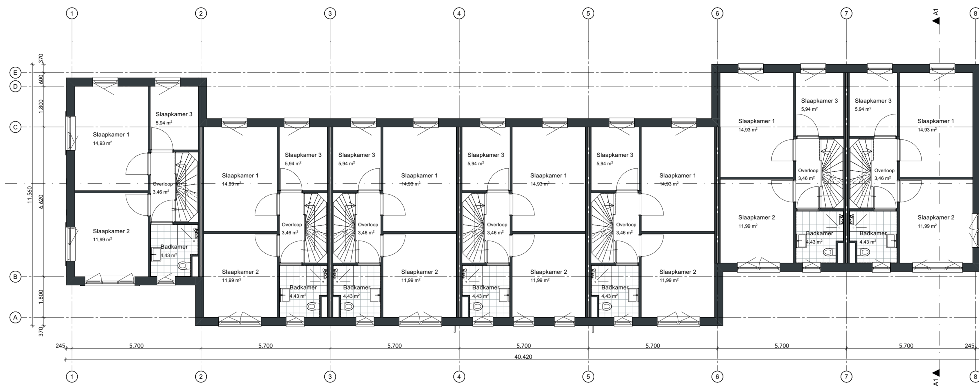
01 eerste verdieping
