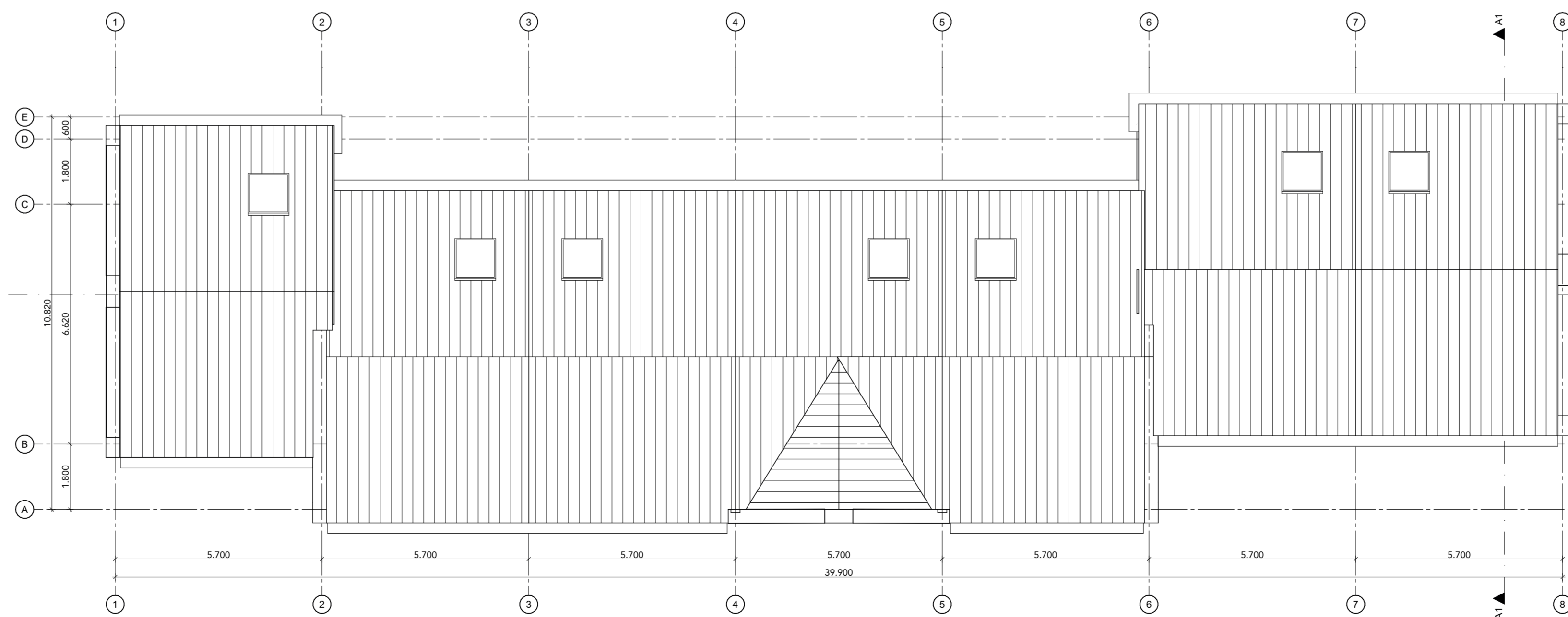
03 dakaanzicht
